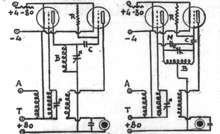
DEUX MONTAGES A RÉSONNANCE
