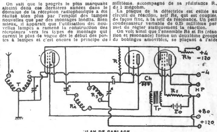
PLAN DE CABLAGE
