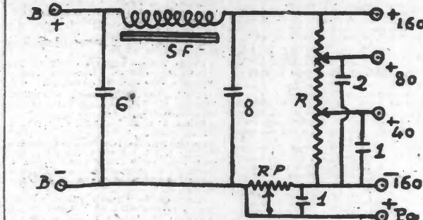
SCHEMA DE FILTRE D'ALIMENTATION
