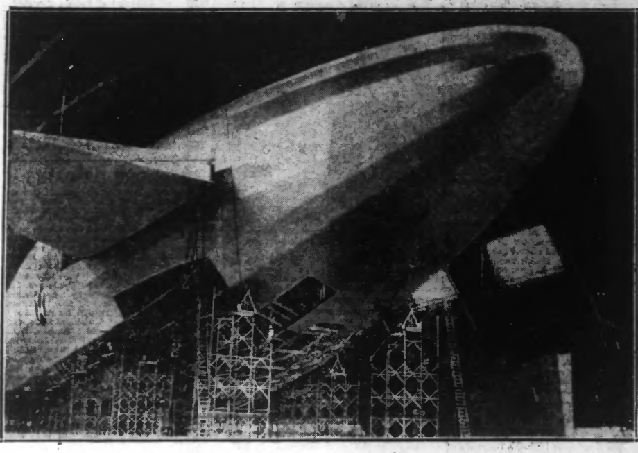
Le « U.S.S. Macon » qu'on est en train de préparer pour ses vols d'essai au printemps prochain, est représenté dans son hangar à Akron (Ohio), où il est en construction pour la marine des Etats-Unis.
