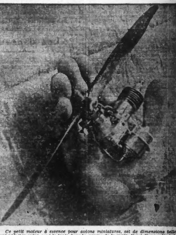
Ce petit moteur à essence pour avions miniatures, est de dimensions tellement réduites qu'on peut le tenir dans la paume de la main. Il est d'une cylindrée de 3 cmc. 5 et tourne à 4.000 tours par minute.
