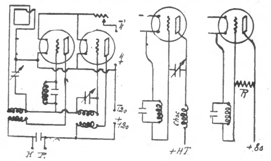
Fig. 1 Réaction électromagnétique, Fig. 2 Réaction électrique par Capacité, Fig. 3 Réaction électrique par résistance.
