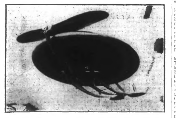
LE NOUVEL APPAREIL EN VOL (Wide World photo.) Un ingénieur italien, M. Guido Talli, a apporté une grande modification au modèle d'avion courant, remplaçant les plans de l'appareil par un disque tournant rempli de gaz.
